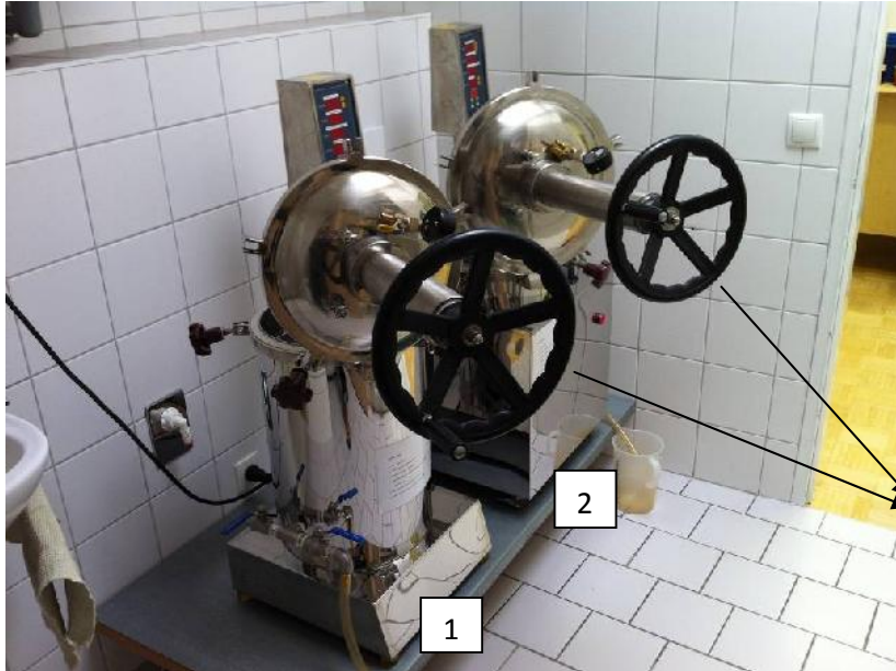
Bild 1: Dekoktmaschinen geöffnet
